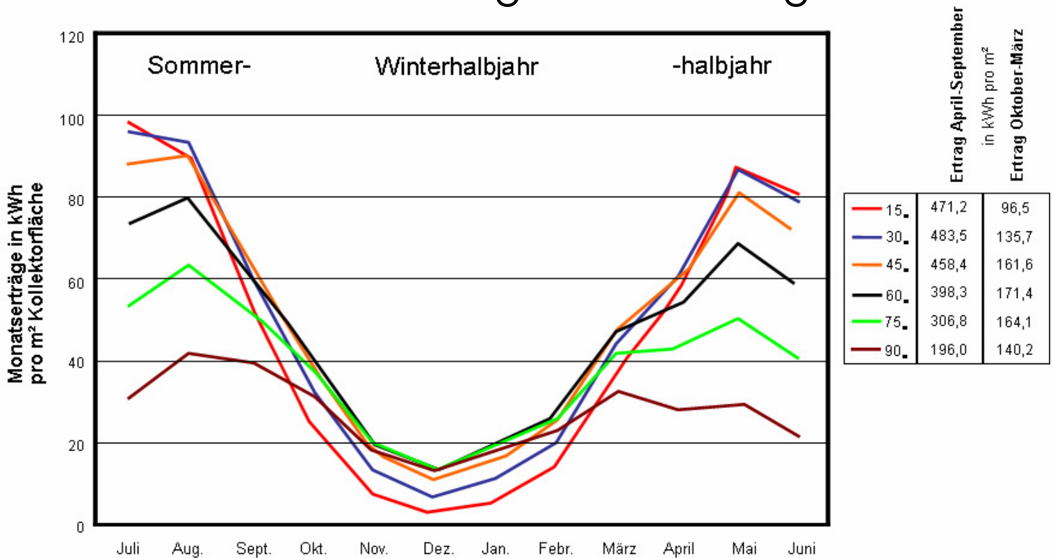
Kollektorsertrag bei fester mittlerer Kollektortemperatur von 40°C in kWh/m 2 ; Standort Stuttgart
